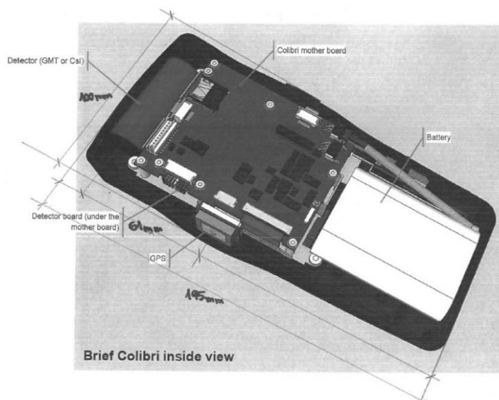
Obr. č. 2 Nákres meradla s rozmermi
